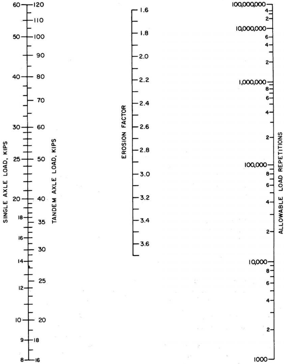
รูปที่ 8 Nomograph สำหรับการวิเคราะห์ Erosion (กรณีมีไหล่ทางคอนกรีต)
