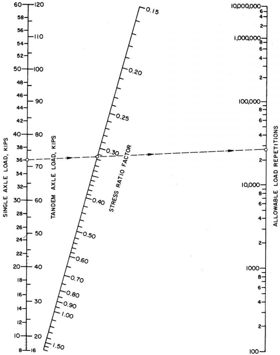
รูปที่ 6 Nomograph สำหรับการวิเคราะห์ Fatigue (กรณีมี และ ไม่มีไหล่ทางคอนกรีต)
