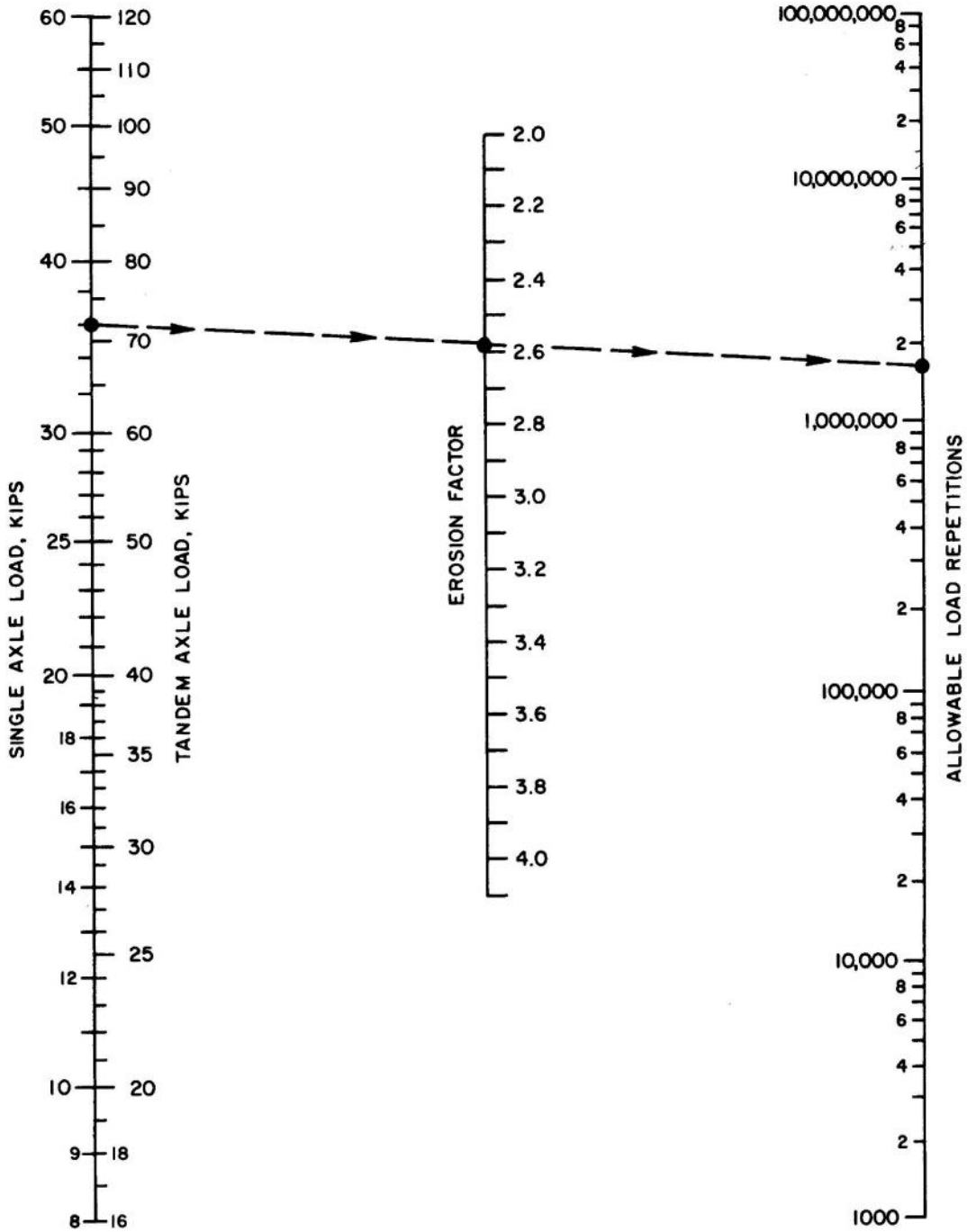
รูปที่ 7 Nomograph สำหรับการวิเคราะห์ Erosion (กรณีไม่มีไหล่ทางคอนกรีต)
